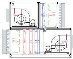
Приточно-вытяжная установка с гликолевым теплоутилизатором (вертикальное исполнение)
