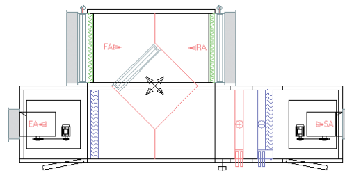
Приточно-вытяжная установка с пластинчатым рекуператором (горизонтальное исполнение)
