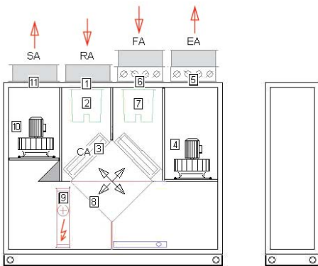
Приточно-вытяжная конфигурация с электрическим нагреванием, тип x40
