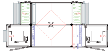
Приточно-вытяжная установка с пластинчатым рекуператором (горизонтальное исполнение)
